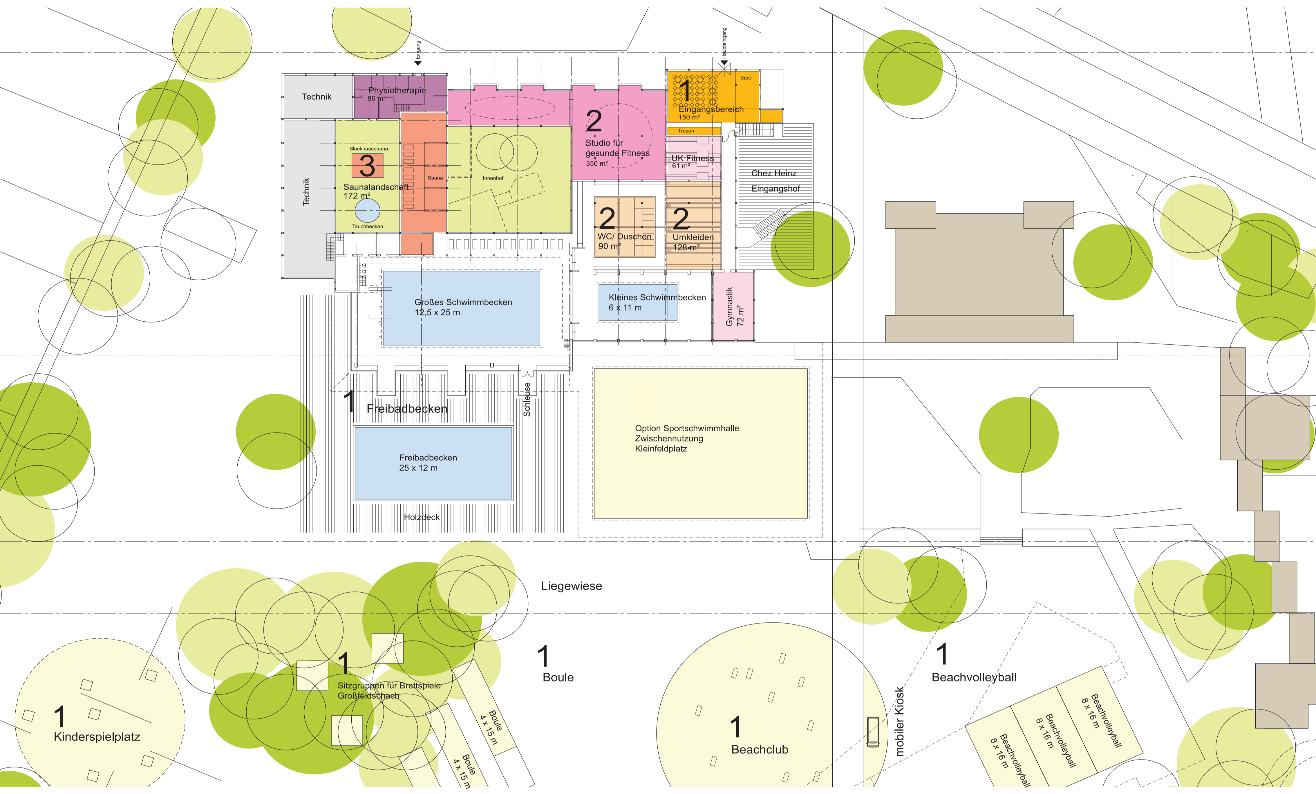
Grundriss _ Ausbaustufe 1-3 _ M. 1 : 500
